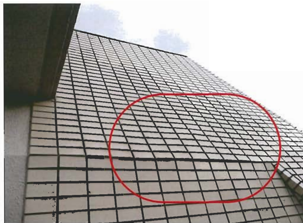
モルタル、タイルの浮き
