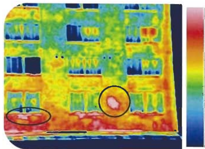
赤外線熱画像
