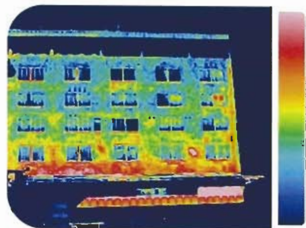
赤外線カメラによる調査 (熱画像による調査・診断)
